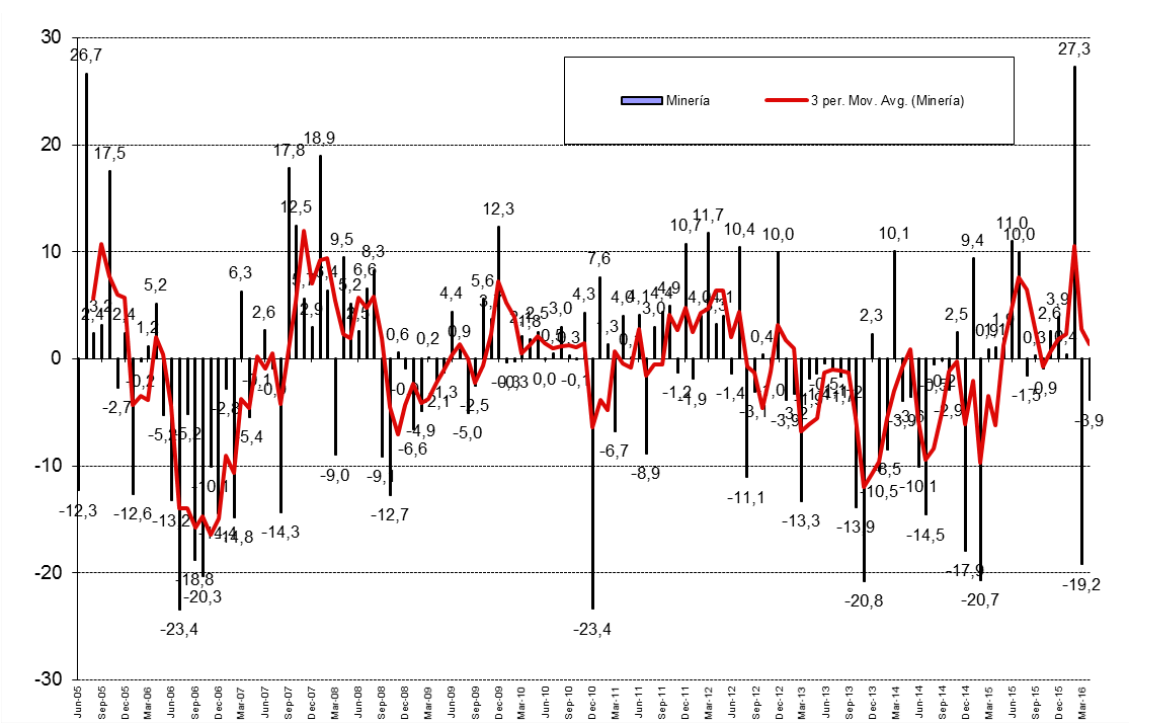
Figura 8. Indicador Difusión del Sector Minería
